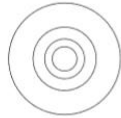
HR 8799
