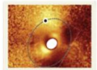
HD 100546b
