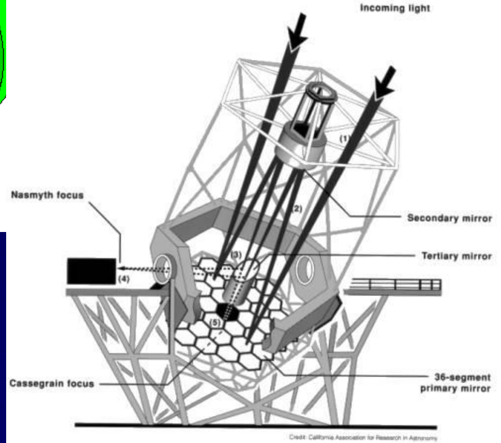
Фокус Нэсмита
