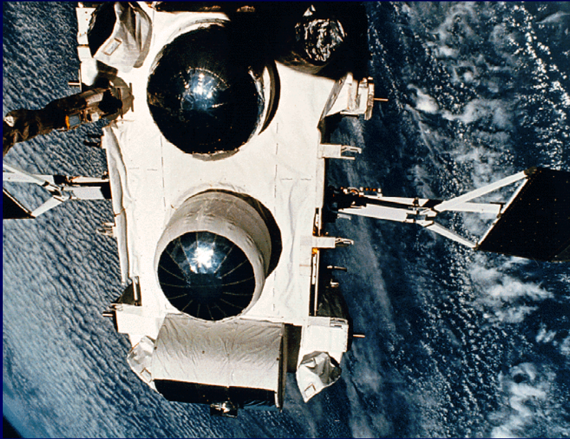
Комптовская гамма обсерватория
