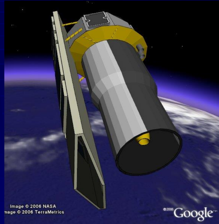
Спитцер
