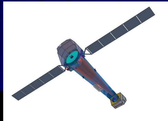
ATHENA (2031)
