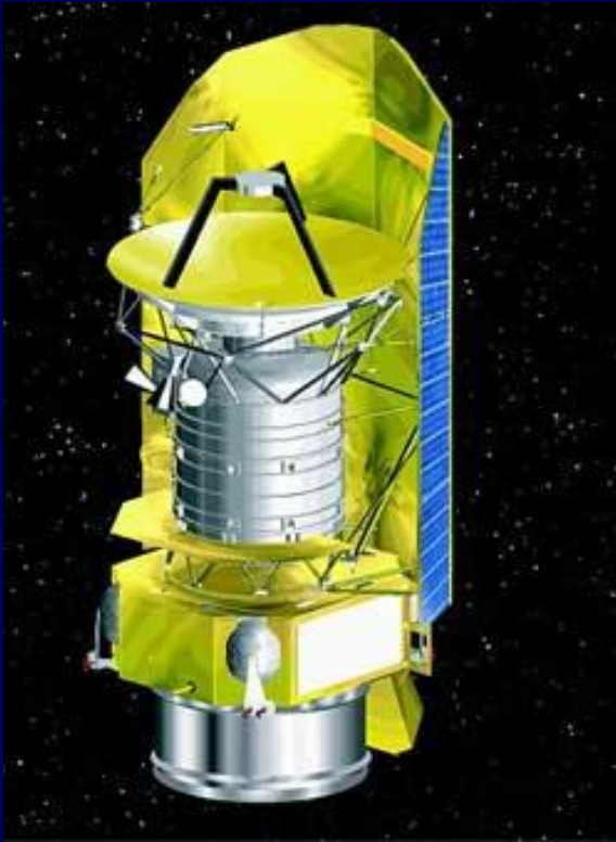
Гершель
