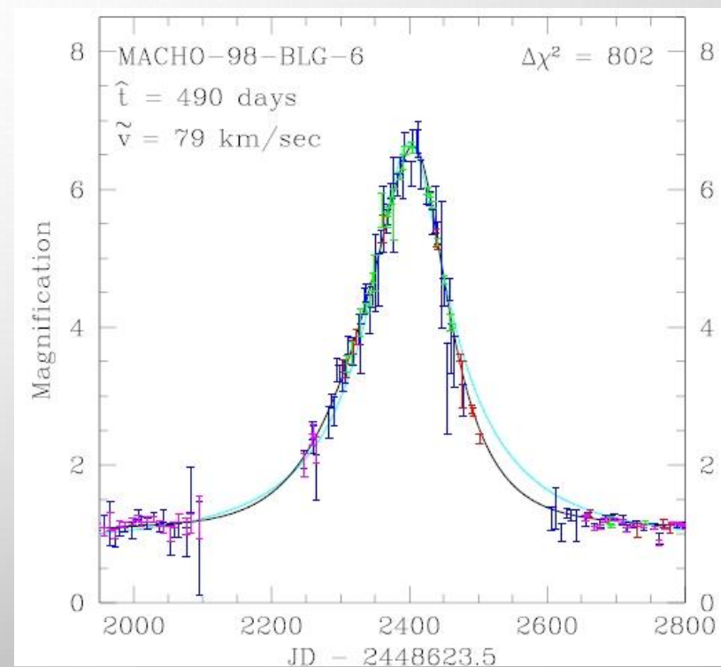
МАСНО-98-BLG-6 3-13 массы Солнца
