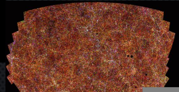
Фон от далеких галактик
