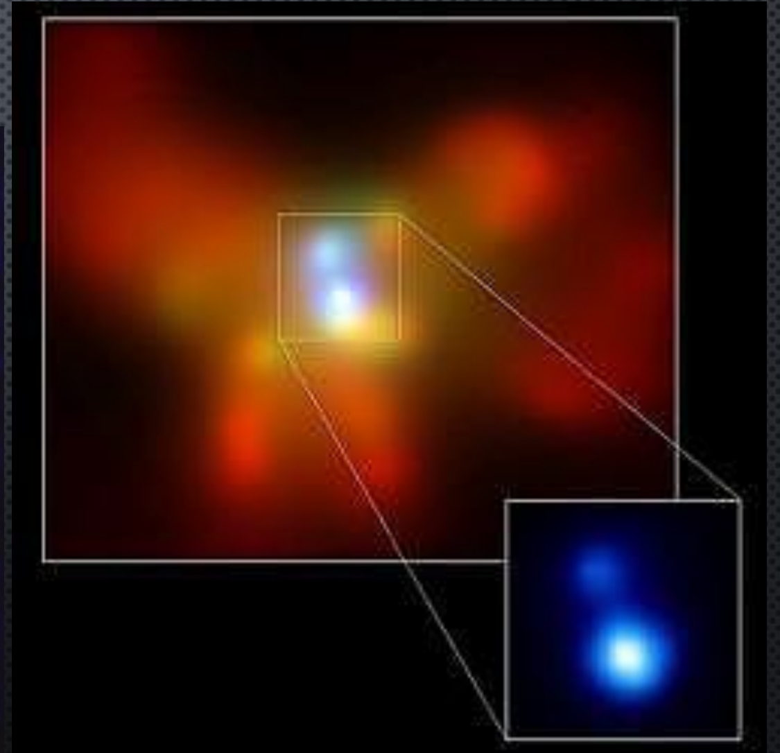
Abell 400
