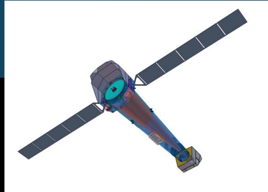
ATHENA (2031)
