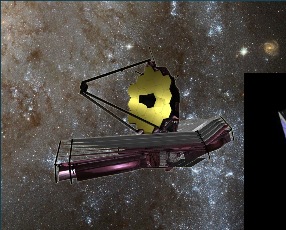
JWST (2022)
