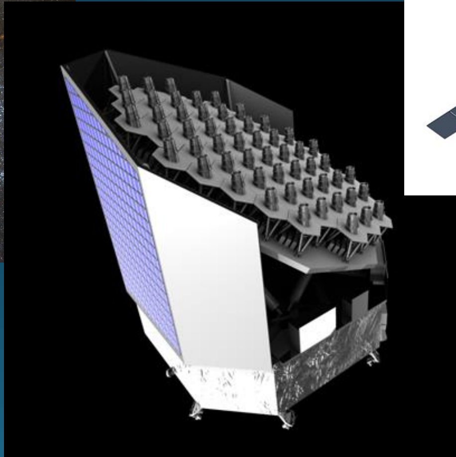
Plato (2026)
